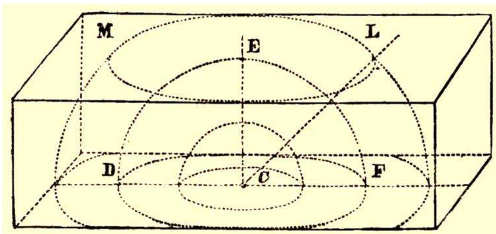
В пособии: Рис. 2.3. С - гипоцентр землетрясения, Е - эпицентр, DEF - сейсмическая волна под поверхностью, ML - область распространения сейсмической волны на поверхности.
