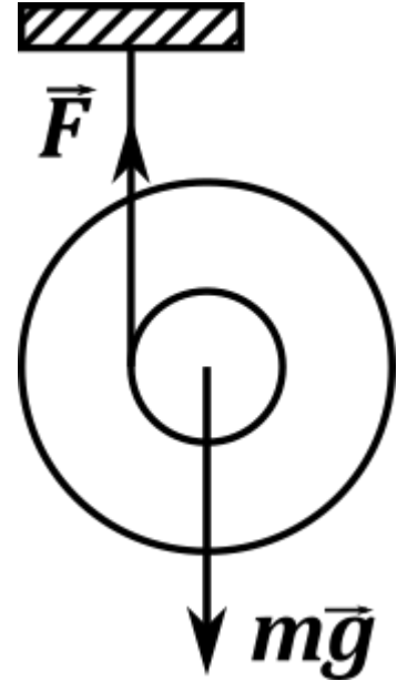
Рис. 1. Схема маятника Максвелла.
