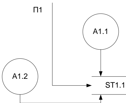
Дочерняя диаграмма 1
