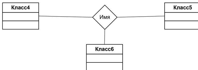
Тернарная ассоциация
