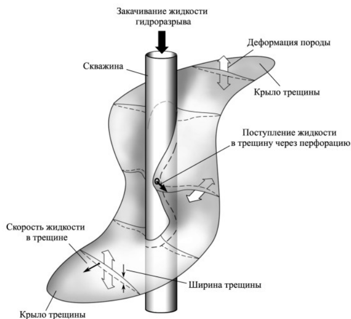
Рис. 1. Схематическая картина процесса гидроразрыва пласта
