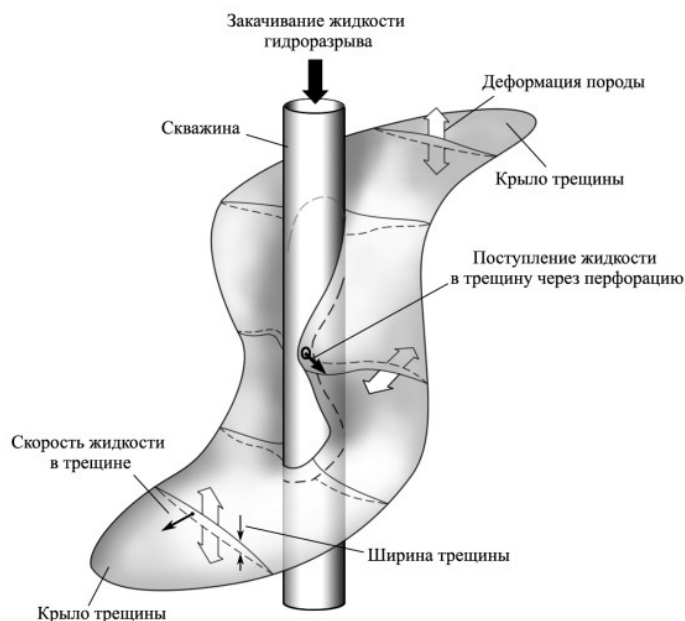
Рис. 1. Схематичная картина процесса гидроразрыва пласта
