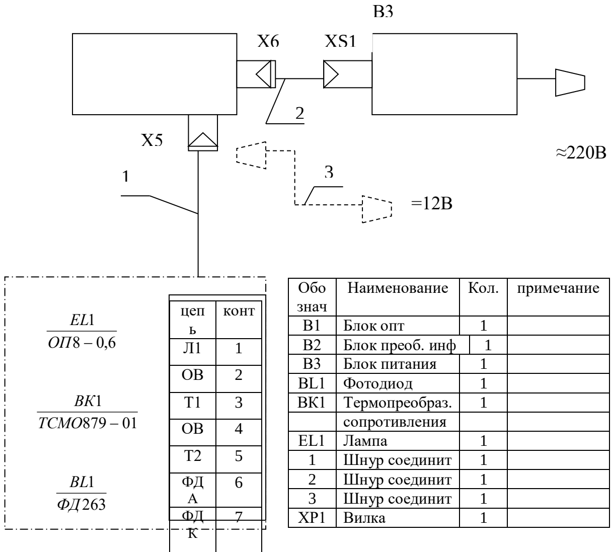
Рис. 1.1 Измеритель переносной. Схема комбинированная общая
