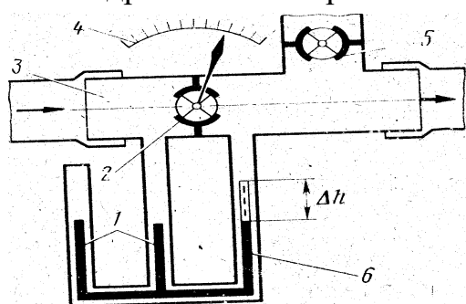
Рис. 4. Схема расходомера ГОСНИТИ КИ-4887-для измерения прорыва газов в картер двигателя.
