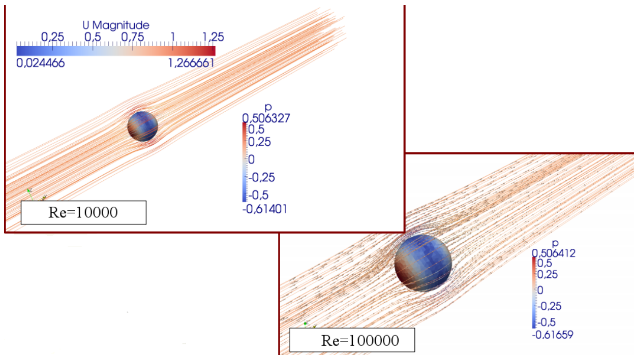
Рис. 67. Примерный вид решения задачи об обтекании сферы.
