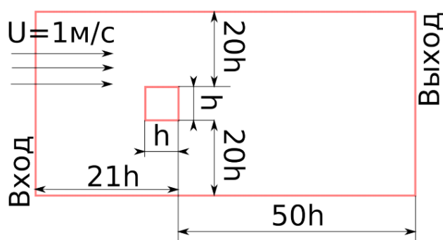
Рис. 47. Условия задачи об обтекании бруса.
