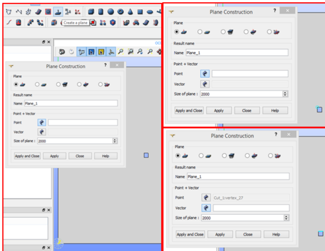
Рис. 52. Построение плоскости.
