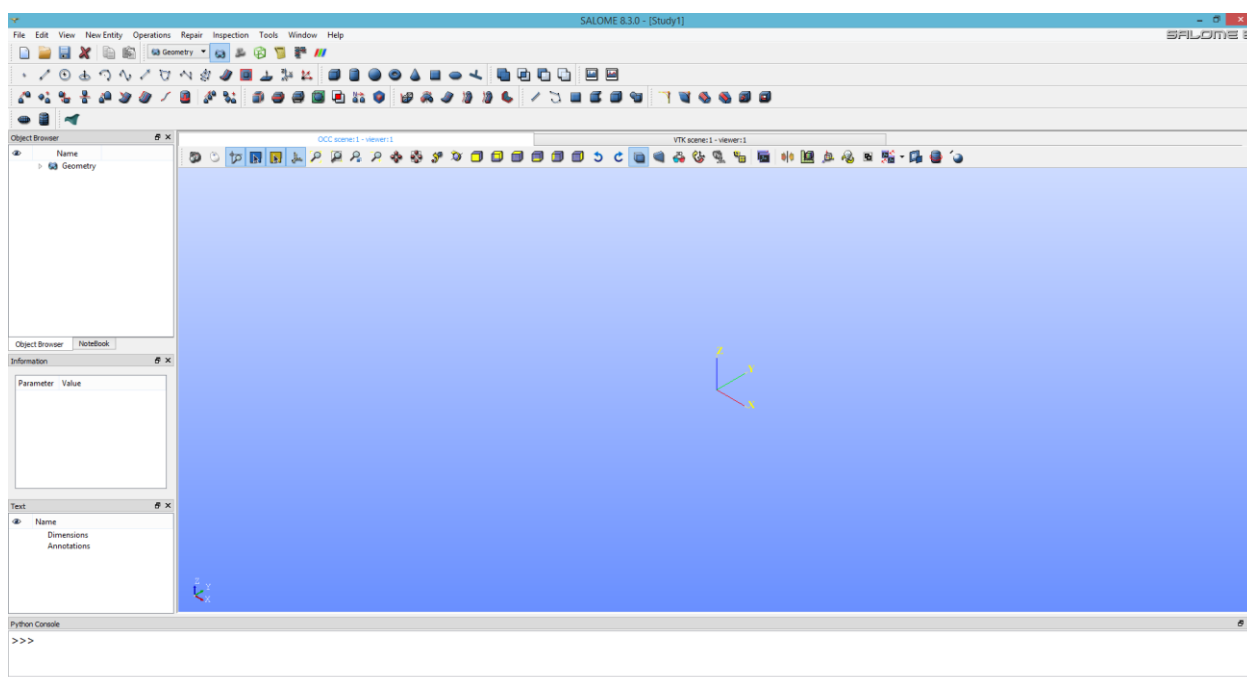
Рис. 9. Интерфейс SALOME.
