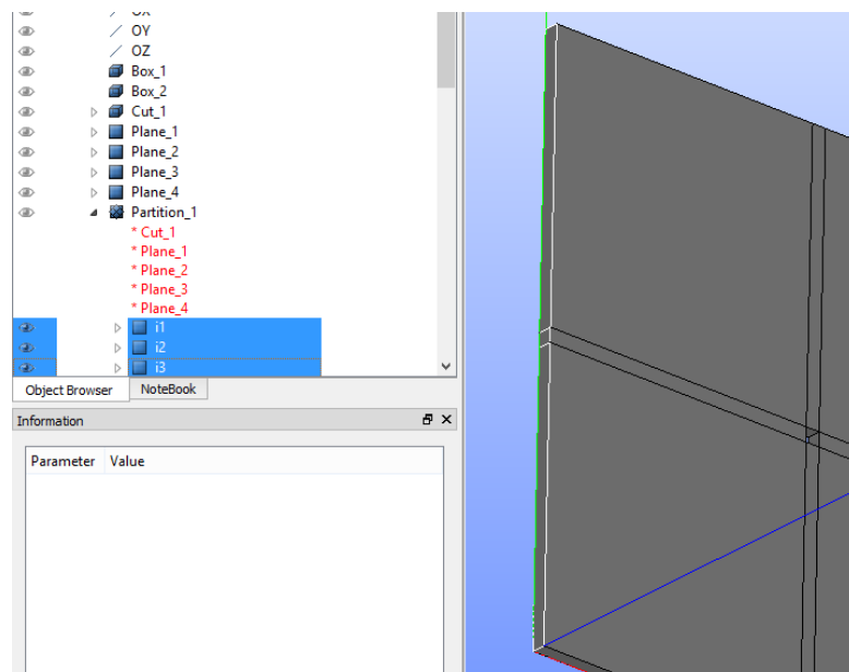
Рис. 58. Переименование поверхностей.
