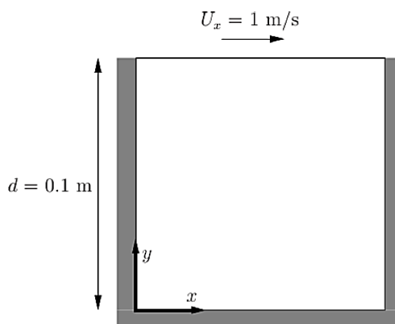
Рис. 10. Схема каверны.
