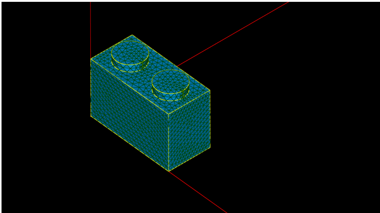
Рис. 34. Разбиение объекта более чем на 14000 элементов.
