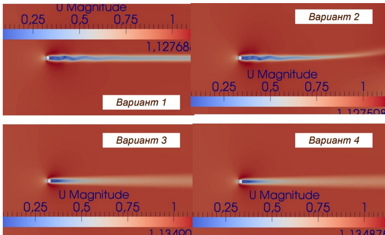
Рис. 61. Примерный вид решения задачи об обтекании бруса.
