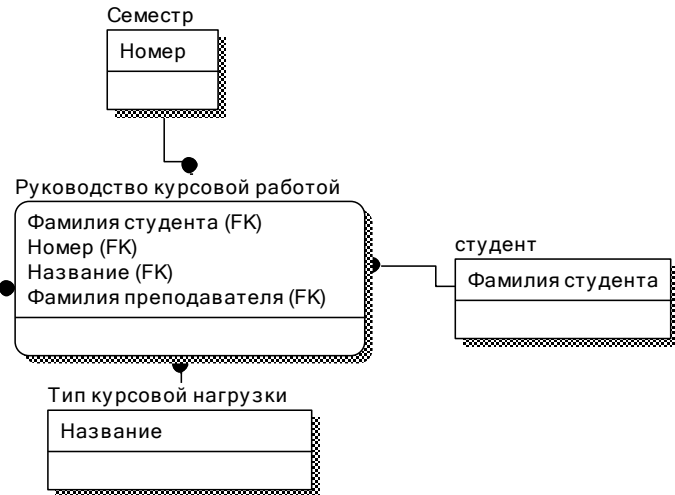
Рисунок 4.27- Удаление сложной связи, за счет введение слабой сущности
