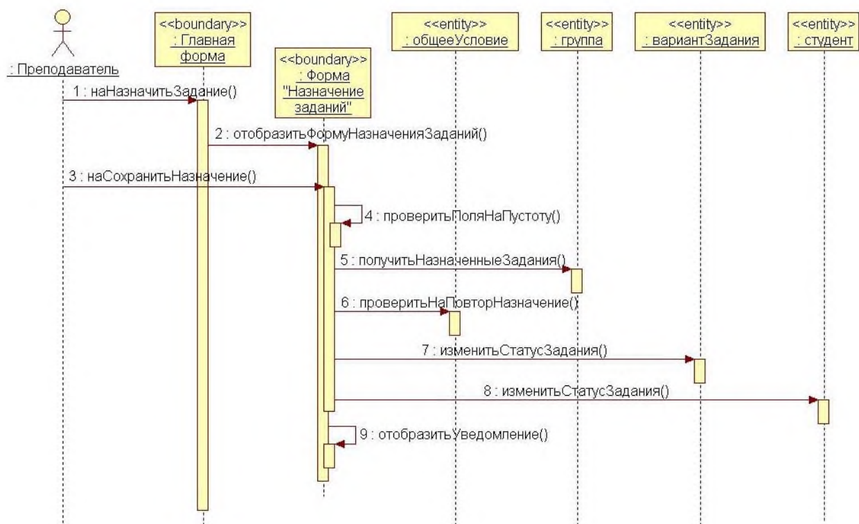
Рисунок 30 – Диаграмма последовательностей для прецедента “Назначить задание студентам”
