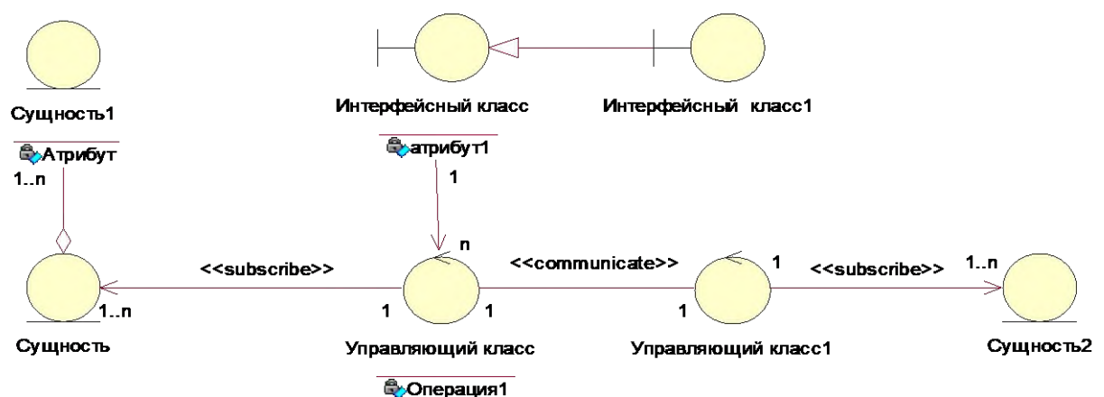
Рисунок 3.10- Пример реализации ВСЕ в диаграмме классов уровня анализа.
