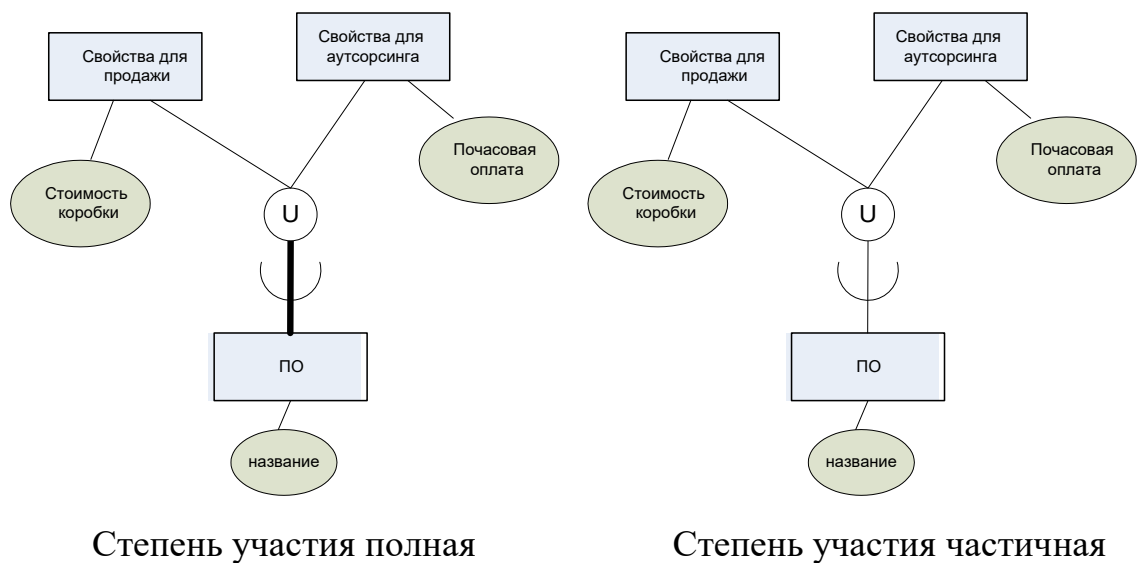
Рисунок 4.18 - Пример использования категории.
