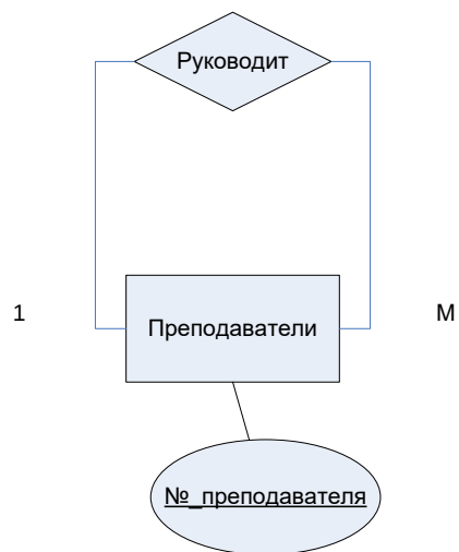
Рисунок 4.28 – Удаление рекурсивной связи
