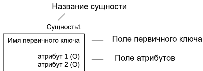
Рисунок 4.19- Сильная сущность
