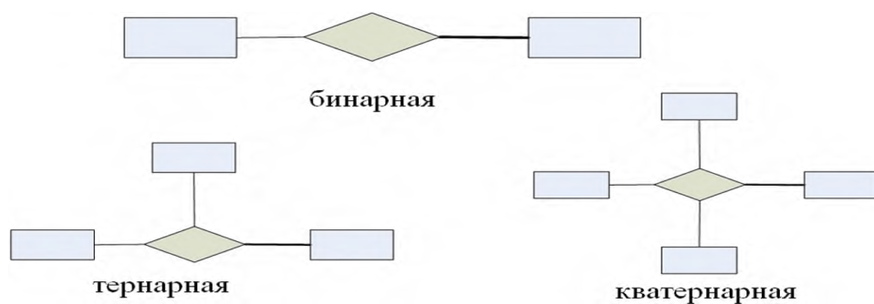
Рисунок 4.14 – Степень связи.
