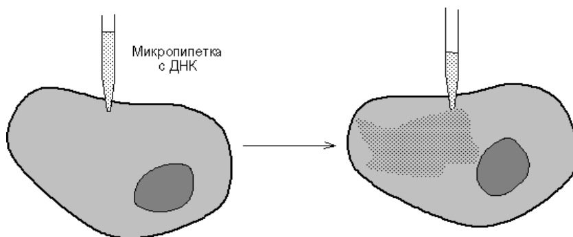
Рис. 23. Микроманипулятор и схема микроинъекции ДНК
