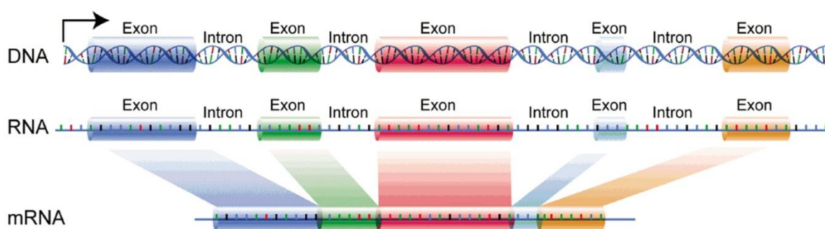
Рис. 11. Процесс сплайсинга
