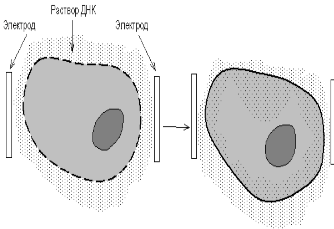
Рис. 13. Процесс электропорации
