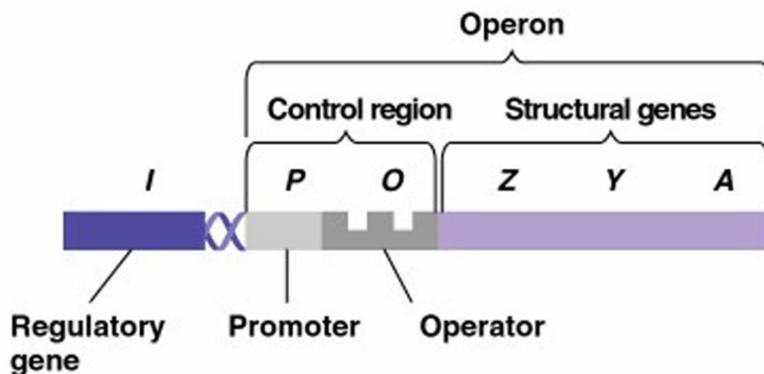
Рис. 10. Структура лактозного оперона
