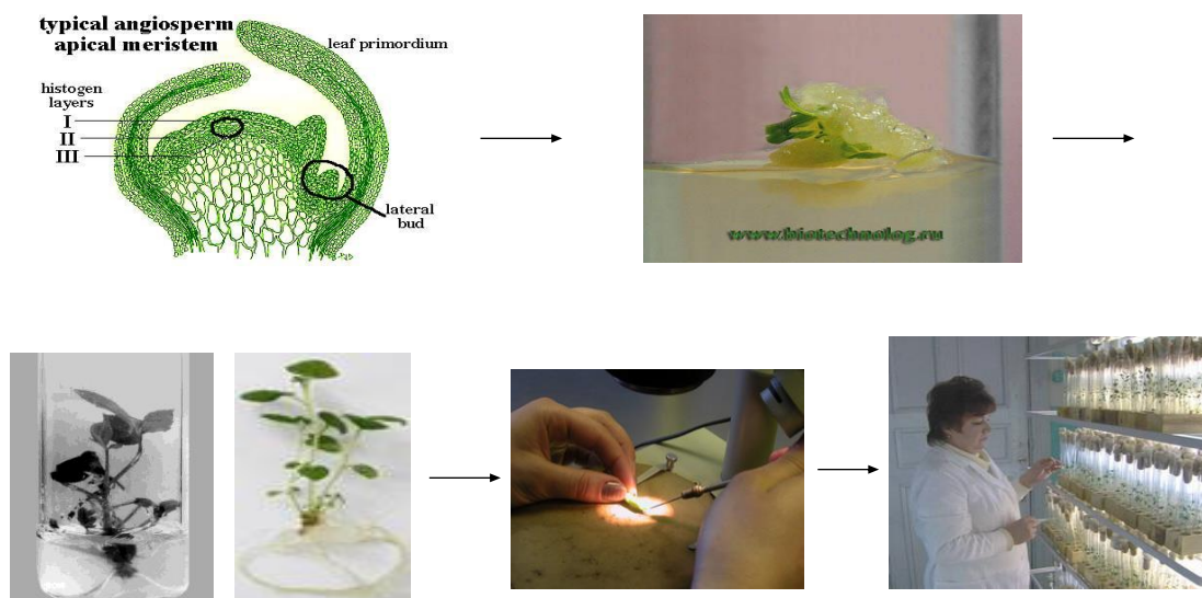
Рис. 25. Технология получения безвирусного картофеля
