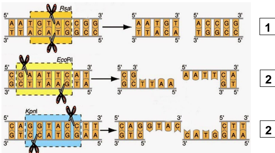
Рис. 8. Расщепление ДНК с образованием «тупых» (1) и «липких» (2) концов
