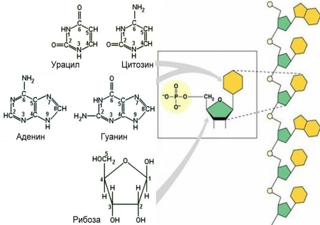
Рис. 3. Структура РНК
