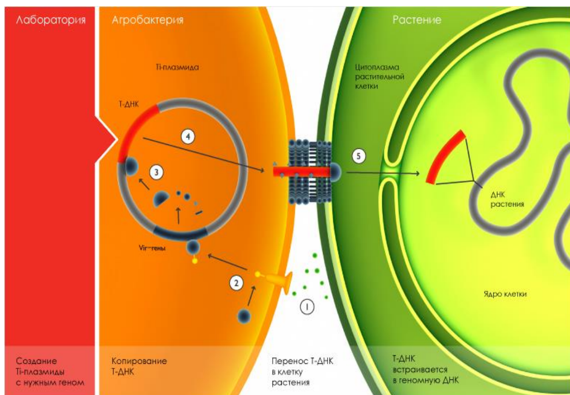
Рис. 27. Встраивание Т-ДНК в геном растения
