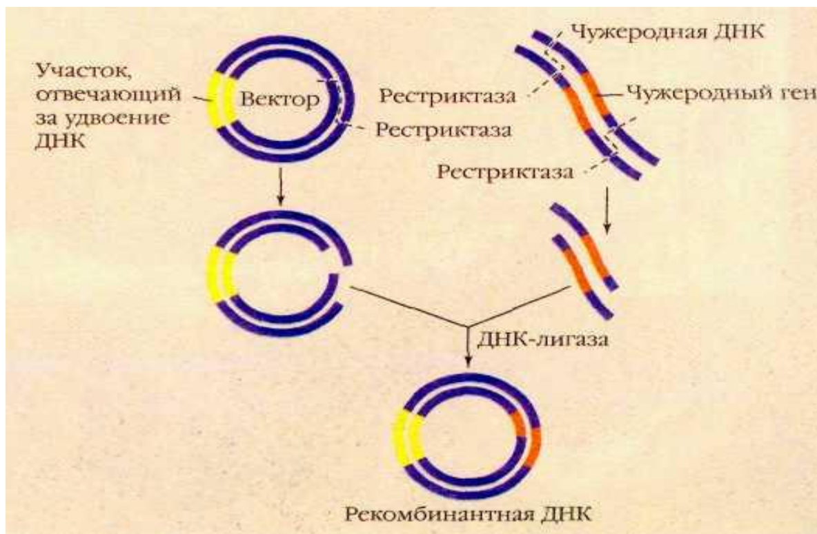
Рис. 5. Создание рекомбинантной ДНК
