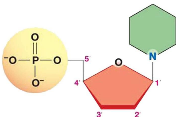
Рис. 1. Структура нуклеотида
