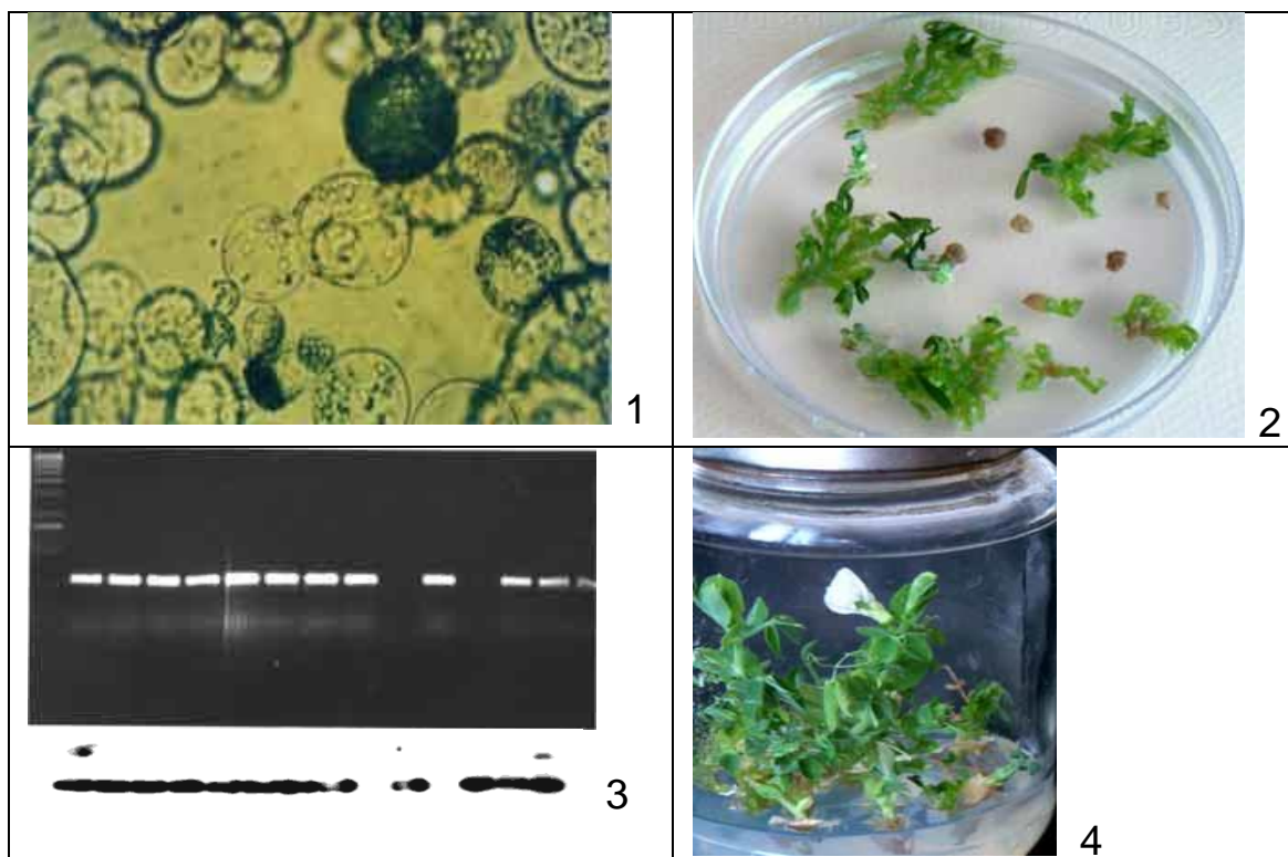
Рис. 29. Этапы трансгенеза
