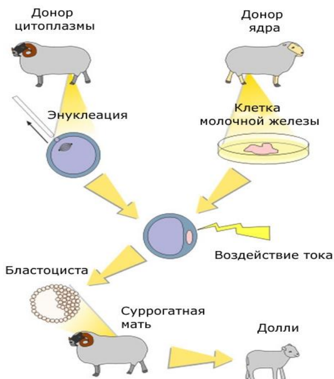
Рис. 22. Создание клонированной овцы
