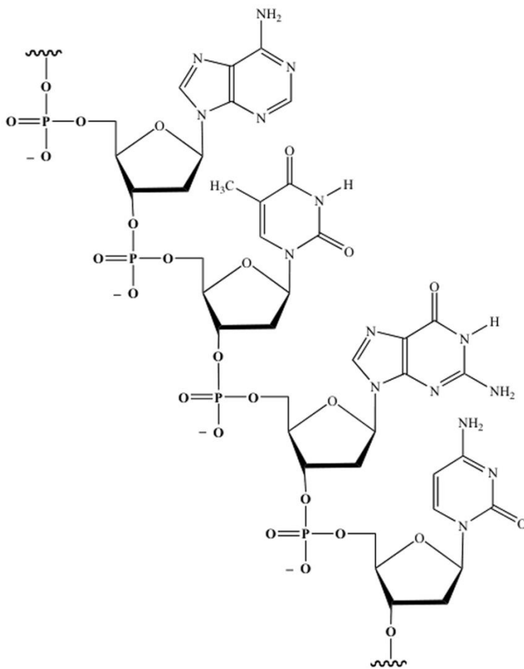
Рис. 2 . Структура ДНК
