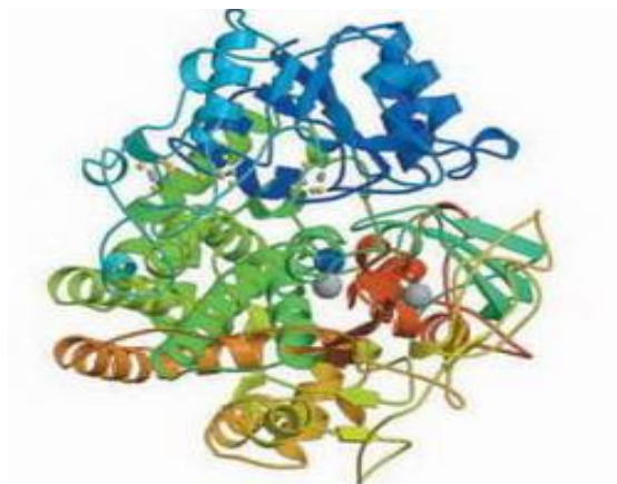
Рис. 6. Структура фермента
