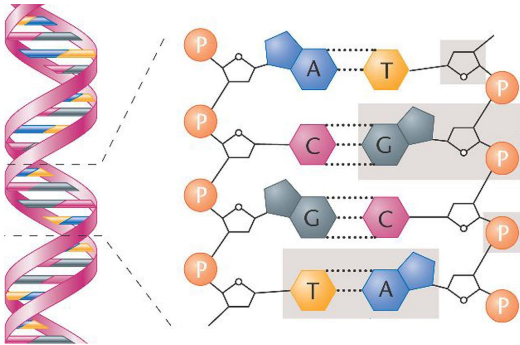
Рис. 4. Принцип комплементарности
