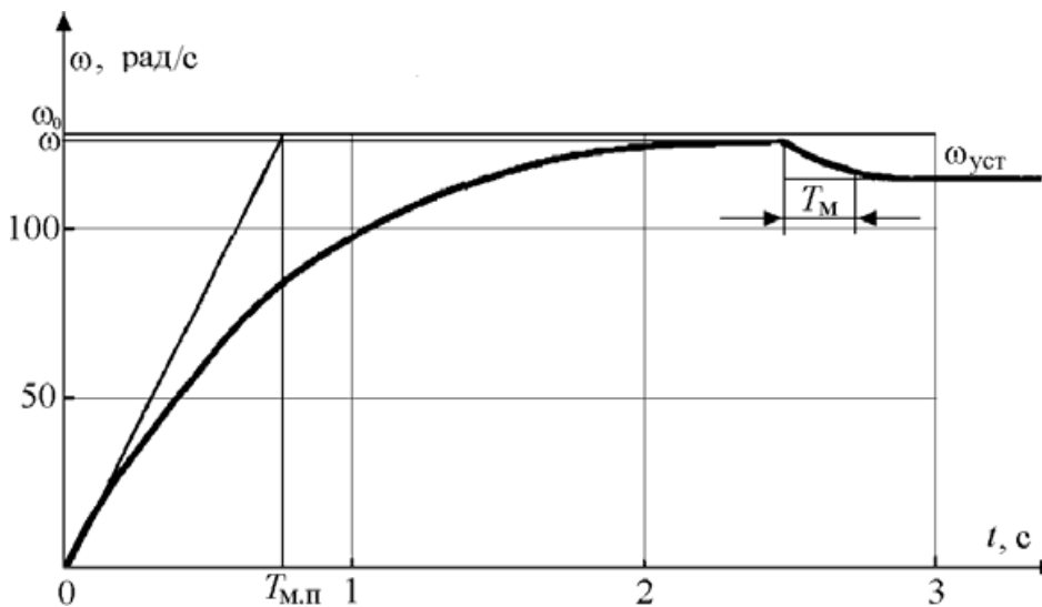
Рис.10. Характеристики при пуске и приложении нагрузки
