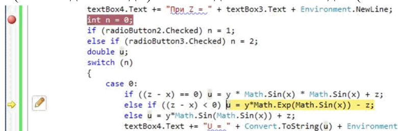
Рис. 4.3. Отладка программы
