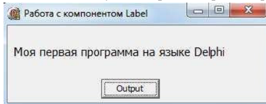
Рисунок 21.4. Окно программы
