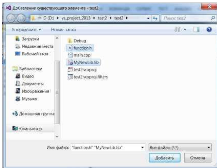
Рисунок 13.5. Выбор функции
