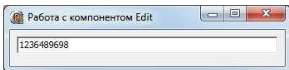
Рисунок 21.11. Готовая программа
