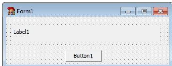
Рисунок 21.1. Форма
