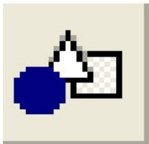
Рисунок 28.1. Компонент Shape
