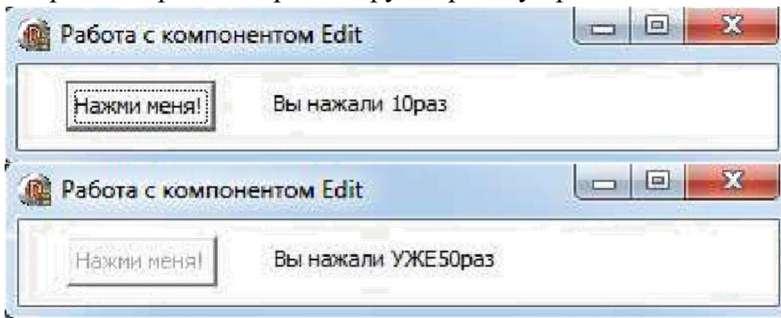
Рисунок 21.18. Готовая программа
