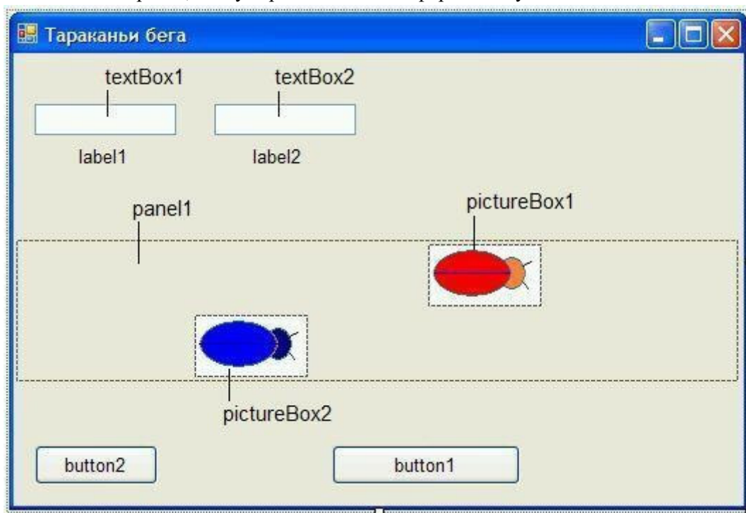
Рисунок 27.2. Форма приложения
