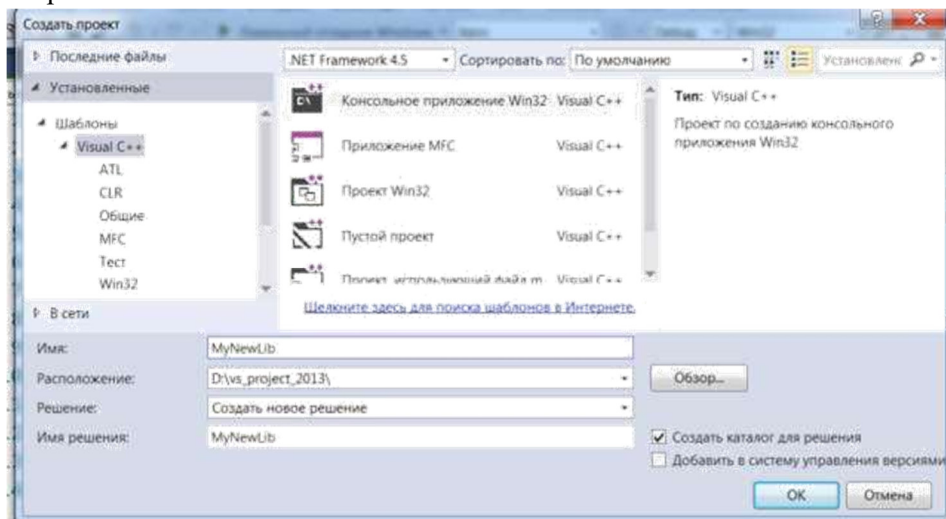
Рисунок 13.1. Создание проекта
