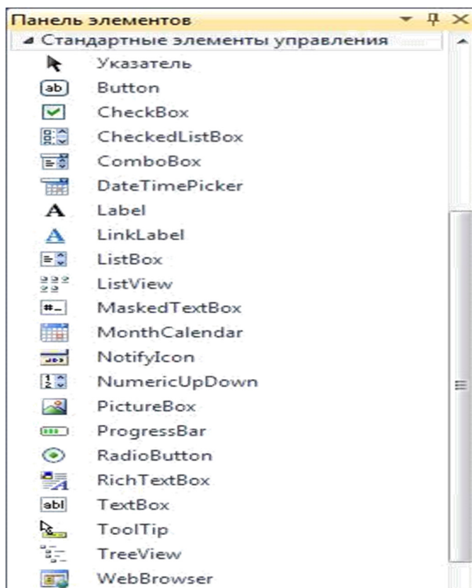
Рис. 1.3. Панель элементов
