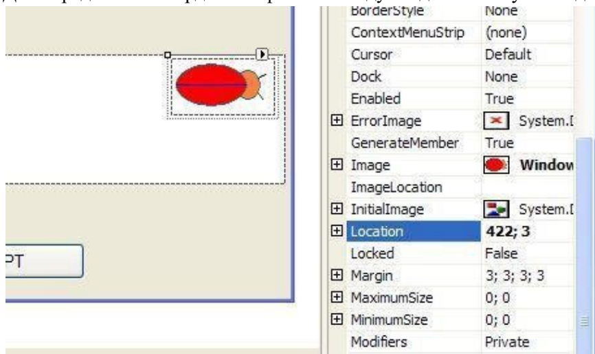
Рисунок 27.5. Настройка координат
