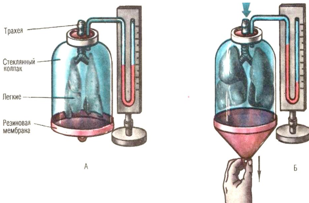
Рис. 19. Опыт Дондерса
