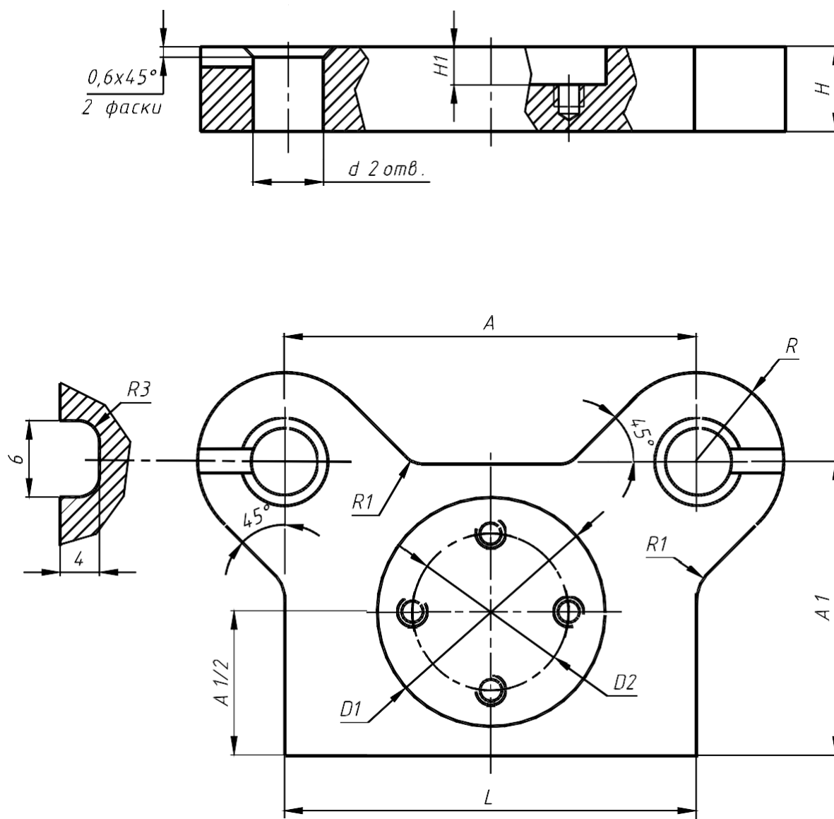
Рис.3. Чертеж с параметрами верхней плиты блока штампа
