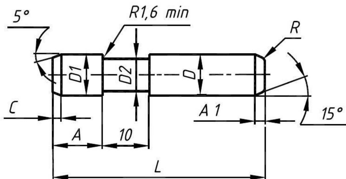
Рис. 5. Чертеж с параметрами ступенчатой колонки блока штампа.
