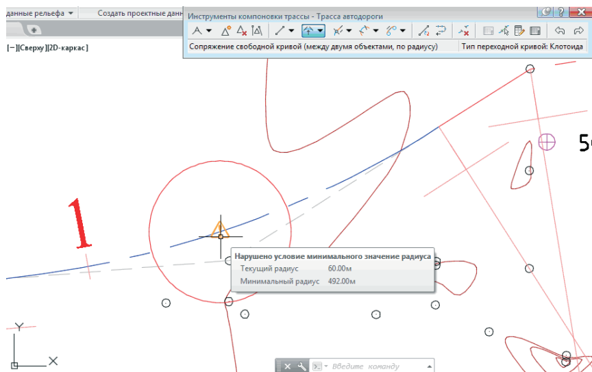
Рис. 7.12. Нарушение условия минимального значения угла
