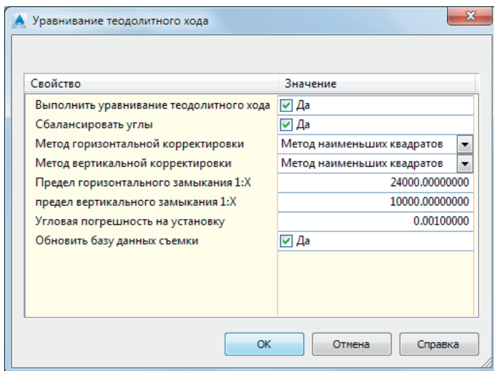
Рис. 4.4. Параметры уравнивания теодолитного хода
