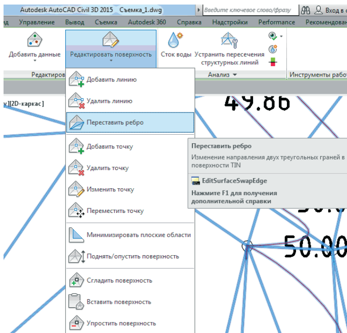
Рис. 5.13. Редактировать поверхность — Переставить ребро
